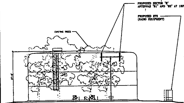
03 SOUTH ELEVATION SCALE: 1/8" = 1'-0"
