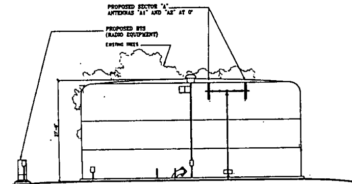
01 NORTH ELEVATION SCALE: 1/8" = 1'-0"
