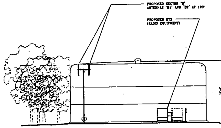
02 EAST ELEVATION SCALE: 1/8" = 1'-0"
