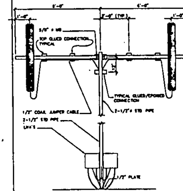
02 ANTENNA SUPPORT SCALE: 1/8" = 1'-0"
