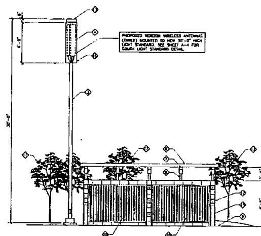
NORTH ELEVATION SCALE: 1/8" = 1'-0"
