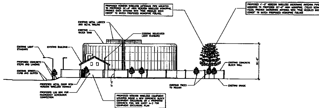
EAST ELEVATION SCALE: 1/8" = 1'-0"
