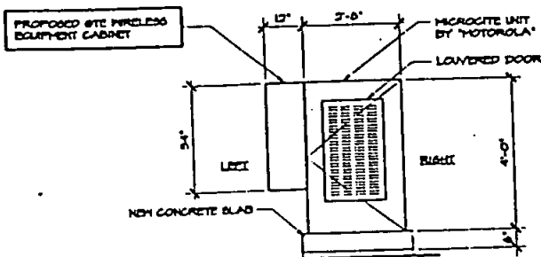
FRONT SIDE ELEVATION SCALE: 1/8" = 1'-0"
