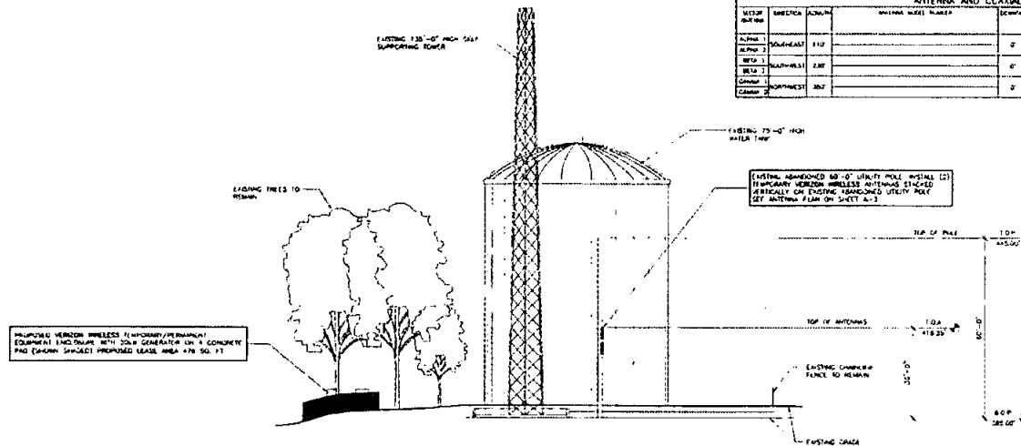
NORTH ELEVATION SCALE: 1/8" = 1'-0"
